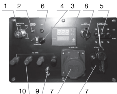
Рис. 3.5 DS 14000 DAC ES
