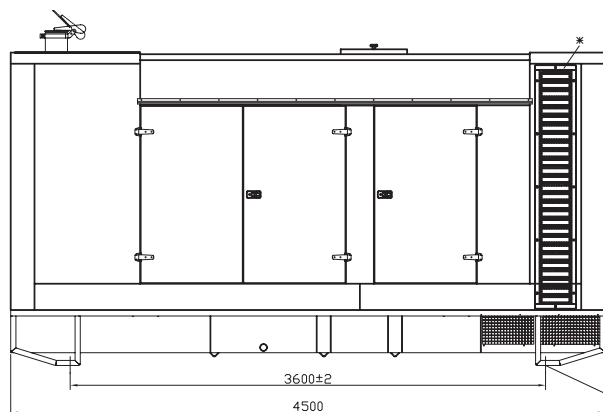
B LATO DESTRO/RIGHT SIDE/ RECHTE SEITE/CÔTÉ DROIT
