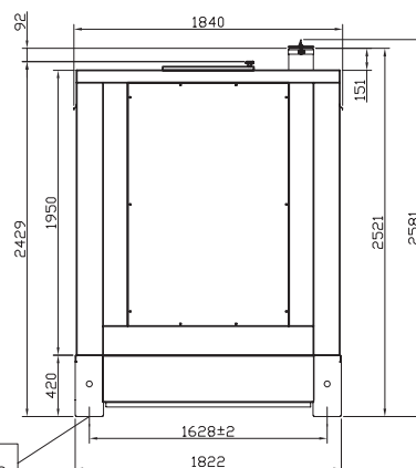
D FRONTE/FRONT/ FRONT/FRONT
