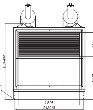
D FRONTE/FRONT/ FRONT/FRONT
