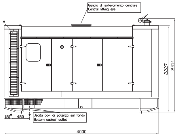
A LATO SINISTRO/LEFT SIDE/ LINKE SEITE/COTE GAUCHE
