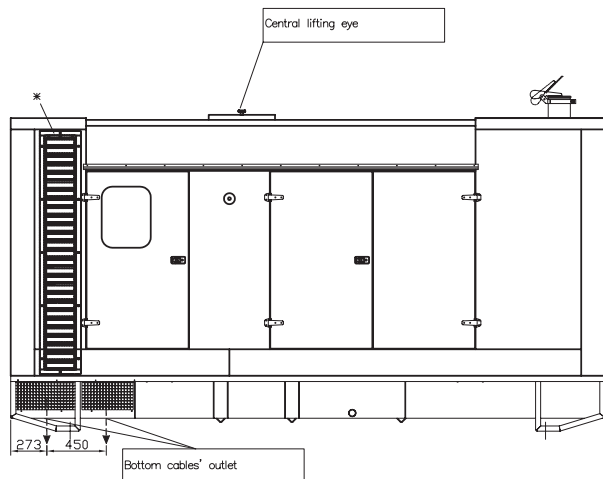
A LATO SINISTRO/LEFT SIDE/ LINKE SEITE/CÔTÉ GAUCHE
