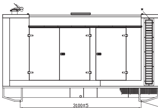
B LATO DESTRO/RIGHT SIDE/ RECHTE SEITE/COTE DROIT
