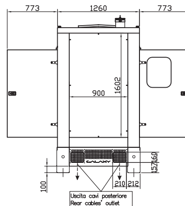
C RETRO/BACK/ RUCKSEITE/DERRIERE
