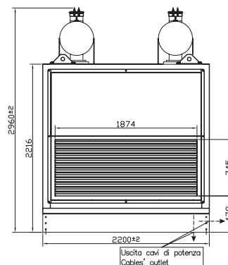
C RETRO/BACK/ RÜCKSEITE/DERRIERE
