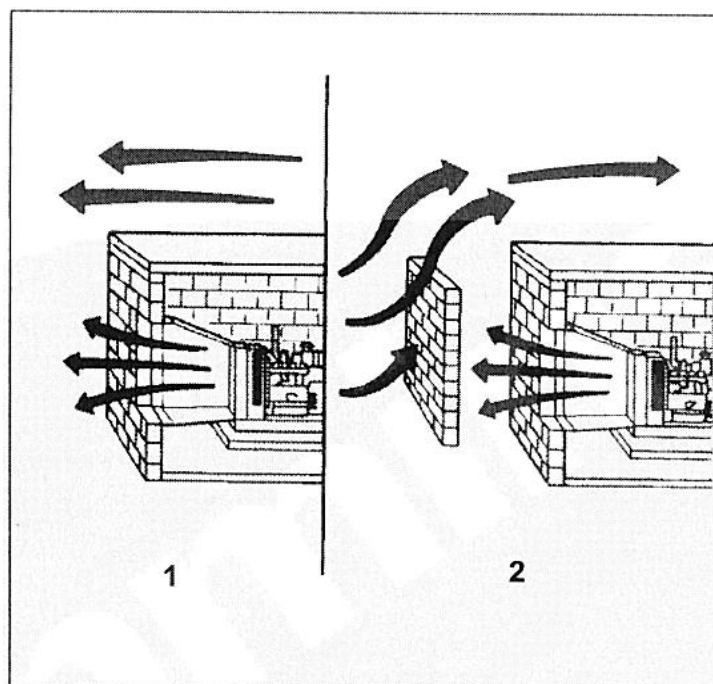
Рис. 10 – Ветрозащитный экран
