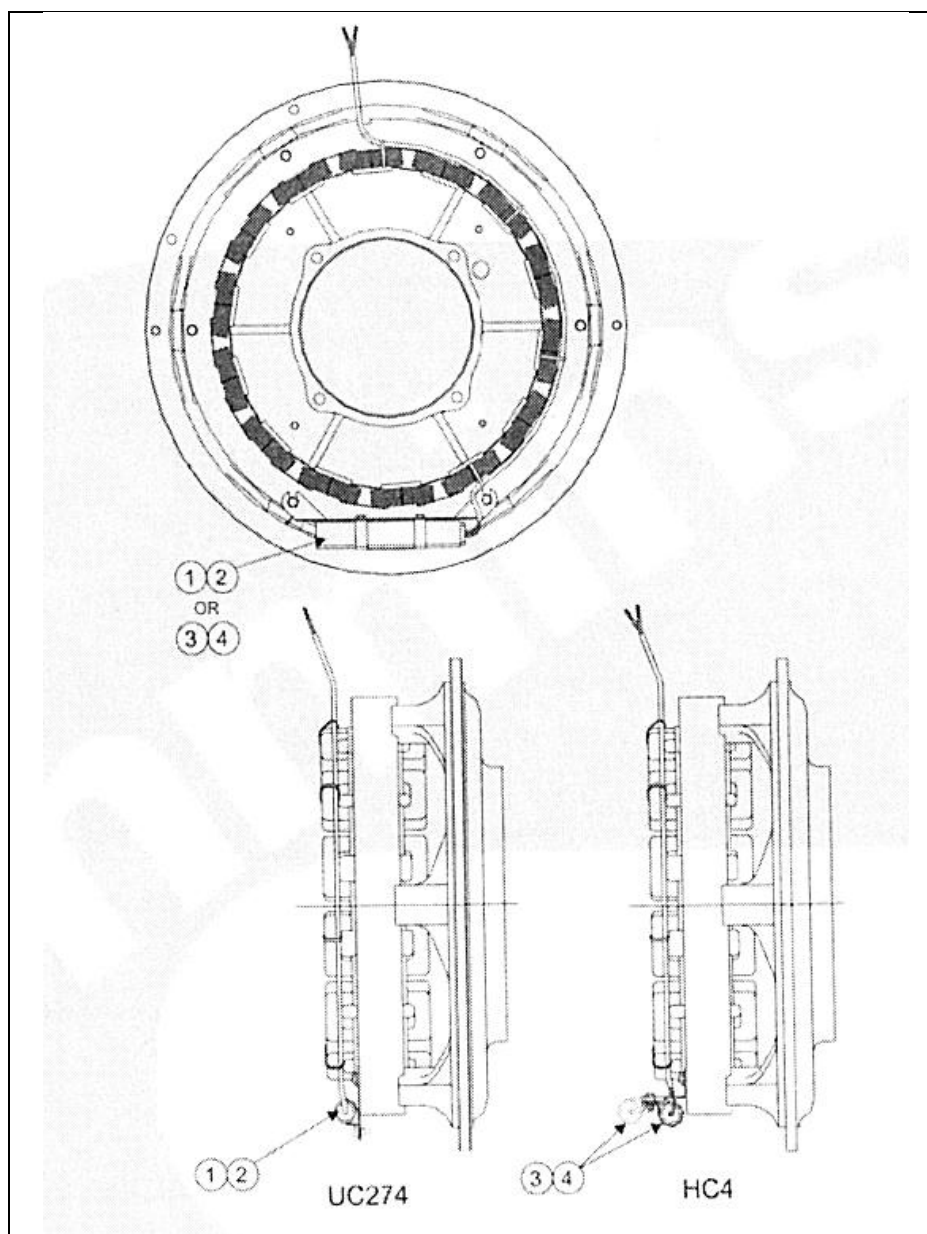
Рис.17 – Подогреватели генератора
